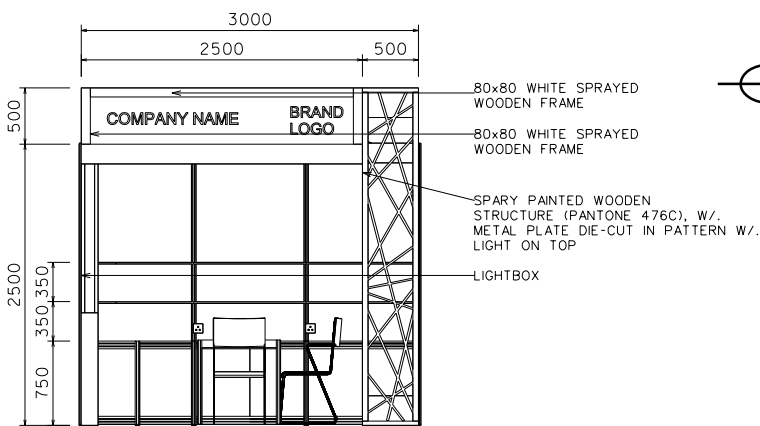
ELEVATION
