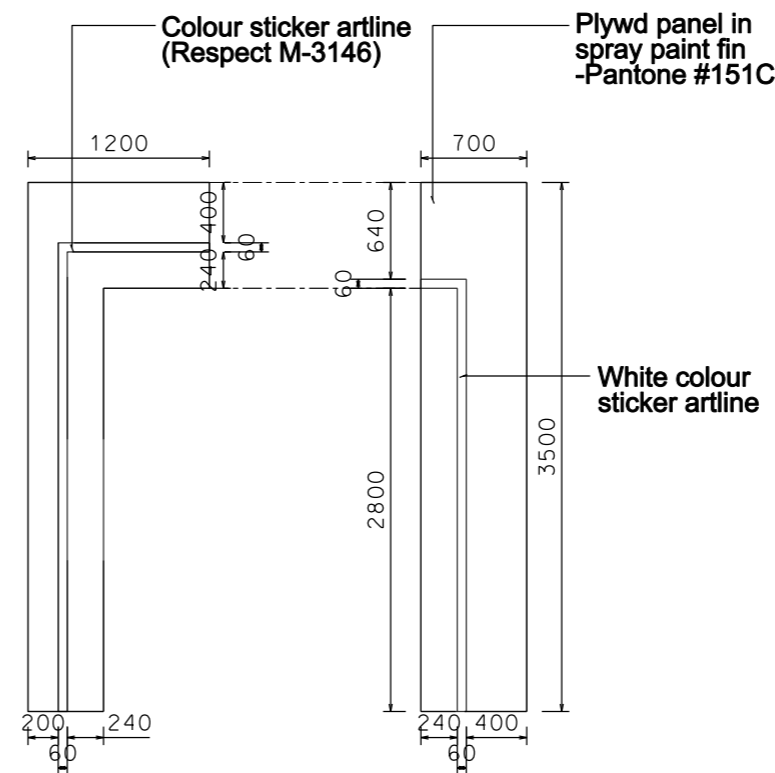
FACSIA ELEVATION
