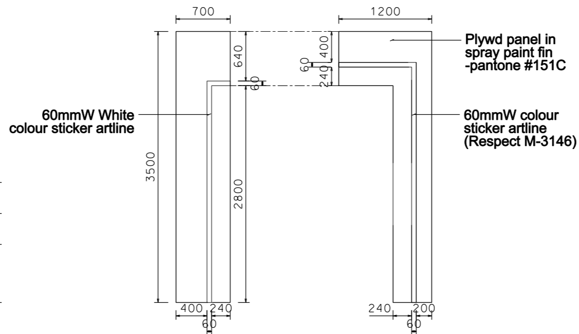
FACIA ELEVATION
