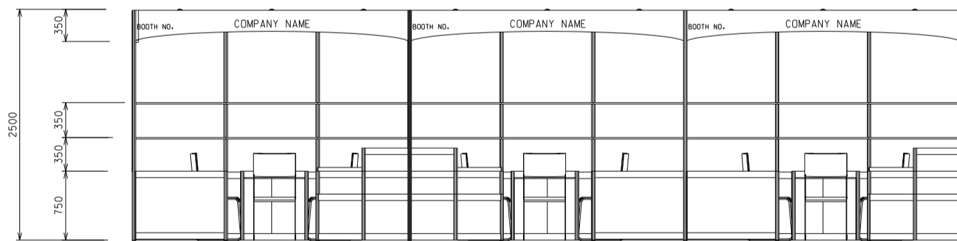
ELEVATION 9M(W) X 3M(D) X 2.5M(H) LEFT CORNER BOOTH B
