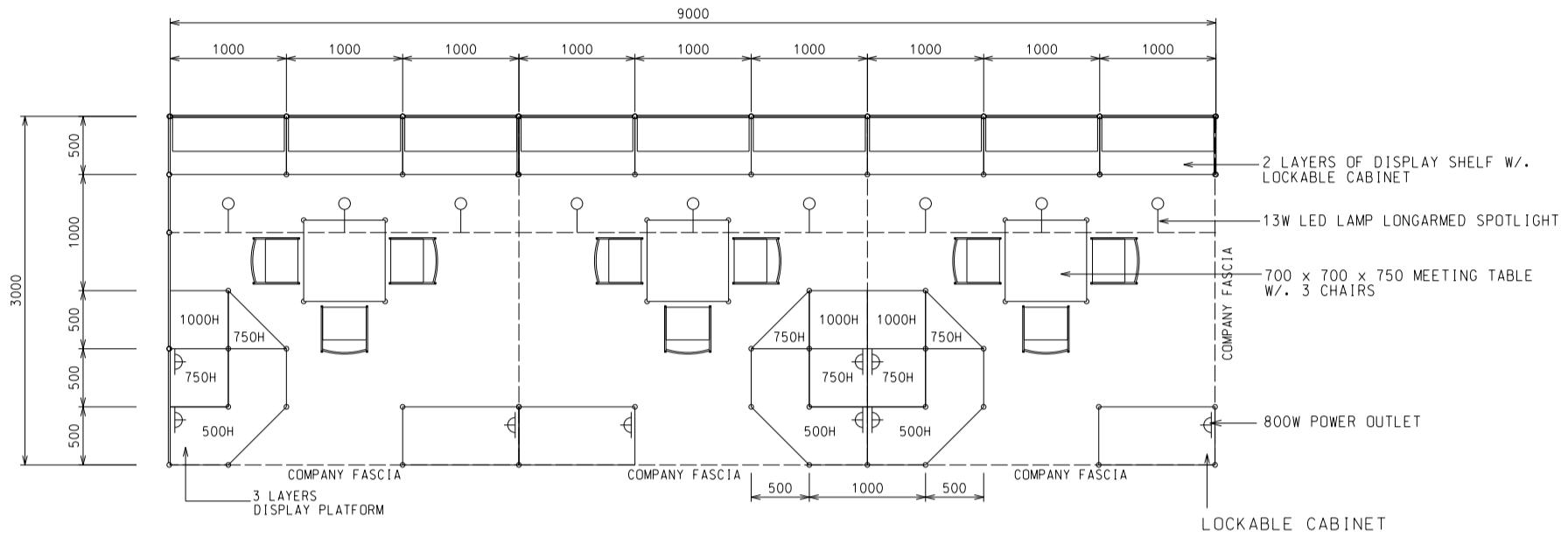
PLAN 9M(W) X 3M(D) X 2.5M(H) RIGHT CORNER BOOTH B
