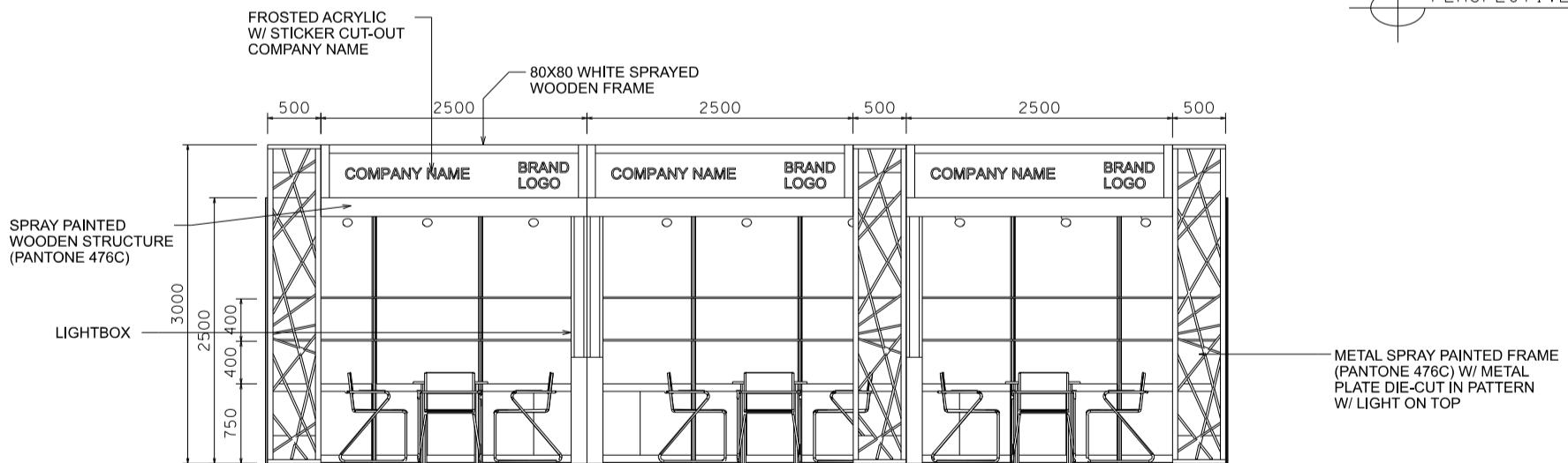
ELEVATION
