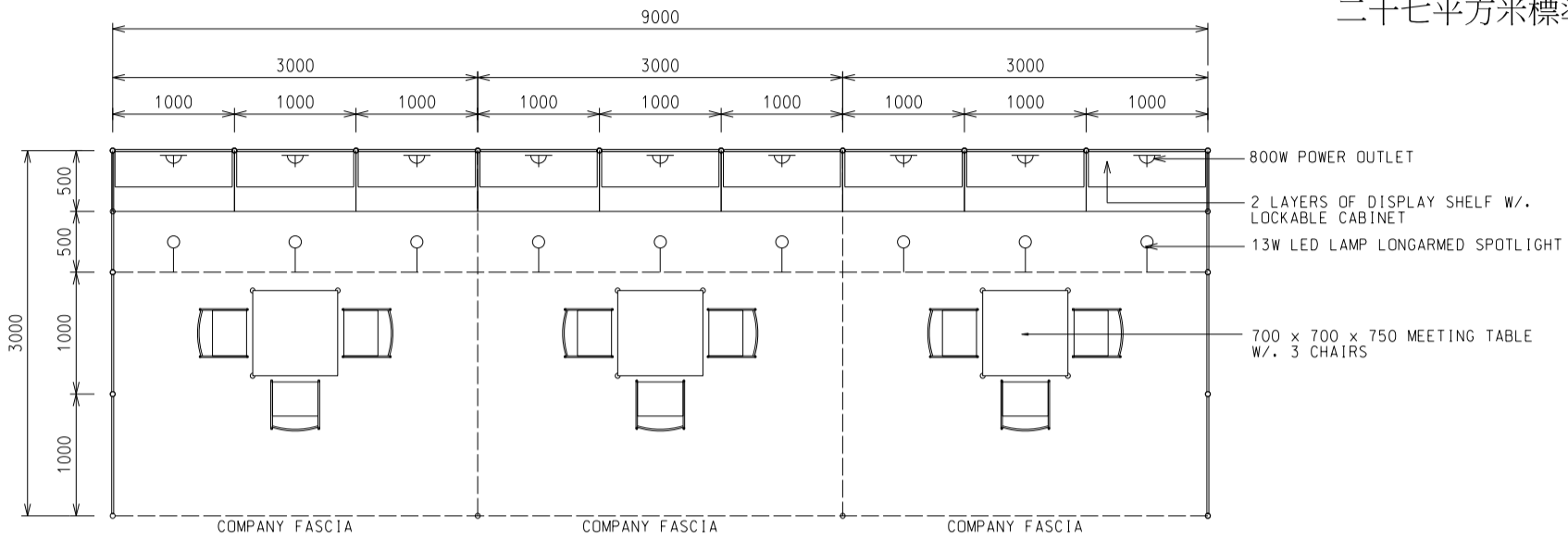
PLAN 9M(W) X 3M(D) X 2.5M(H) Standard Booth A
