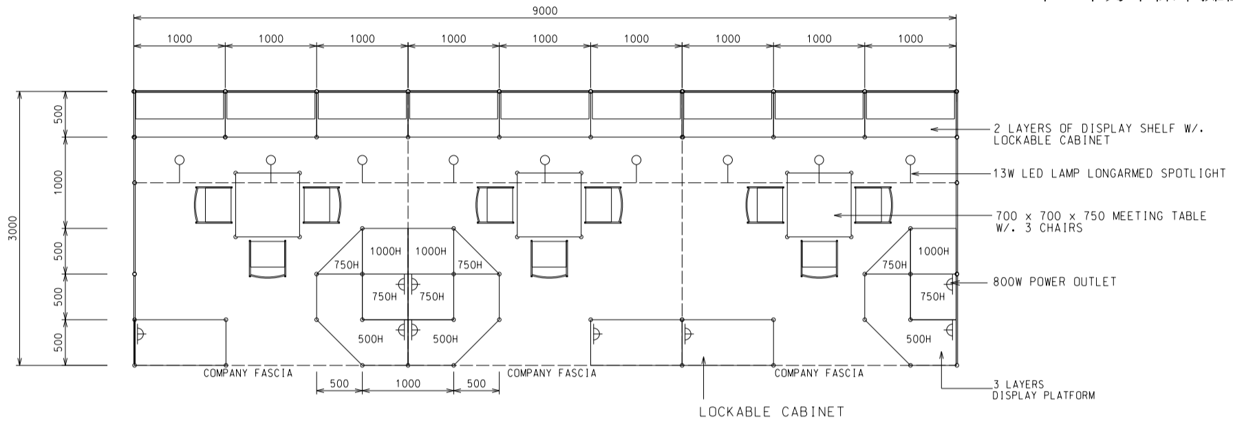
PLAN 9M(W) X 3M(D) X 2.5M(H) STANDARD BOOTH B
