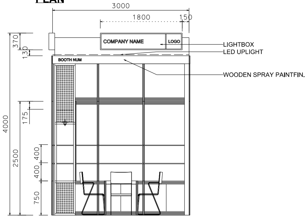
ELEVATION
