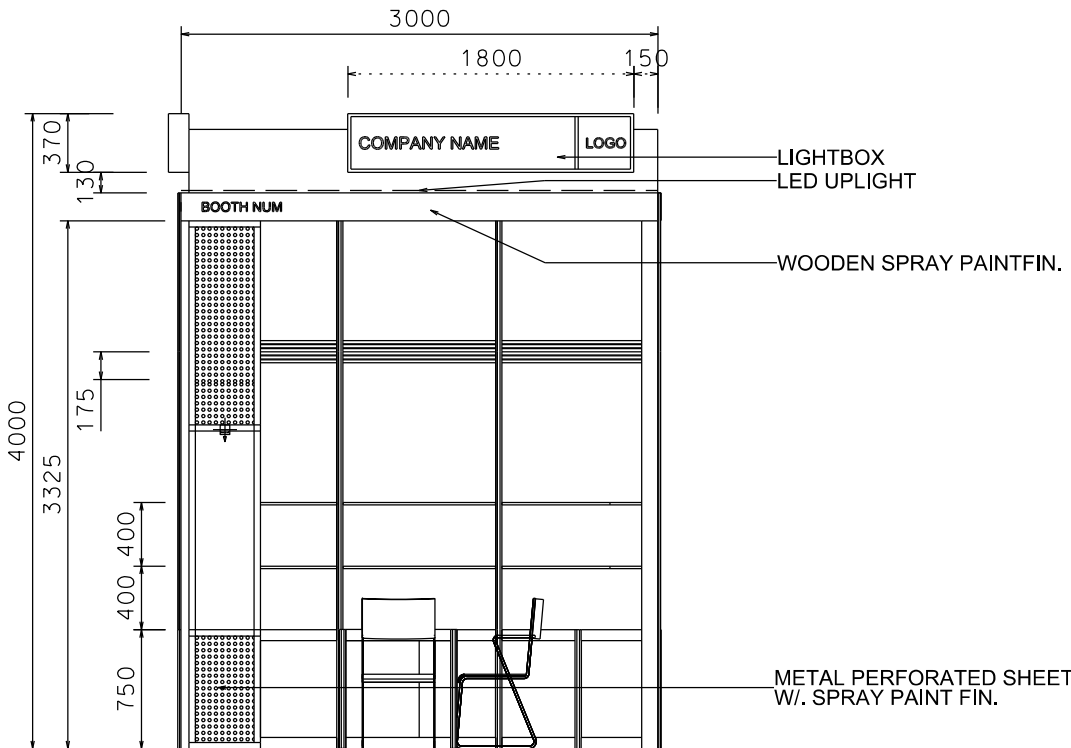
ELEVATION
