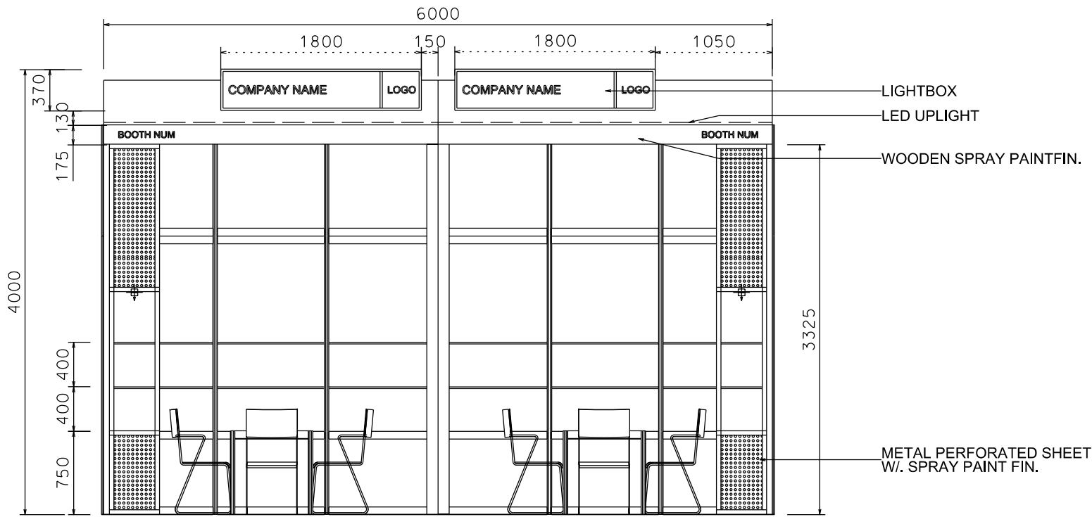
ELEVATION
